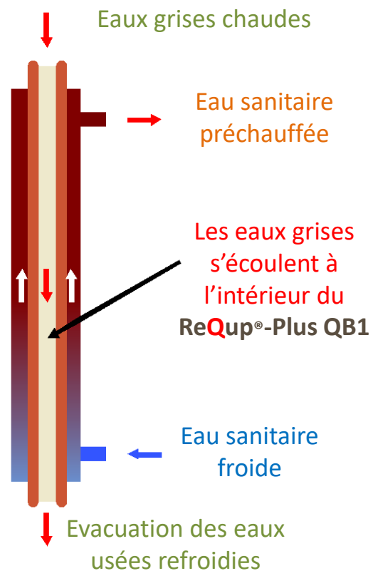
Fig. 2 Coupe longitudinale ReQup-Plus QB1
