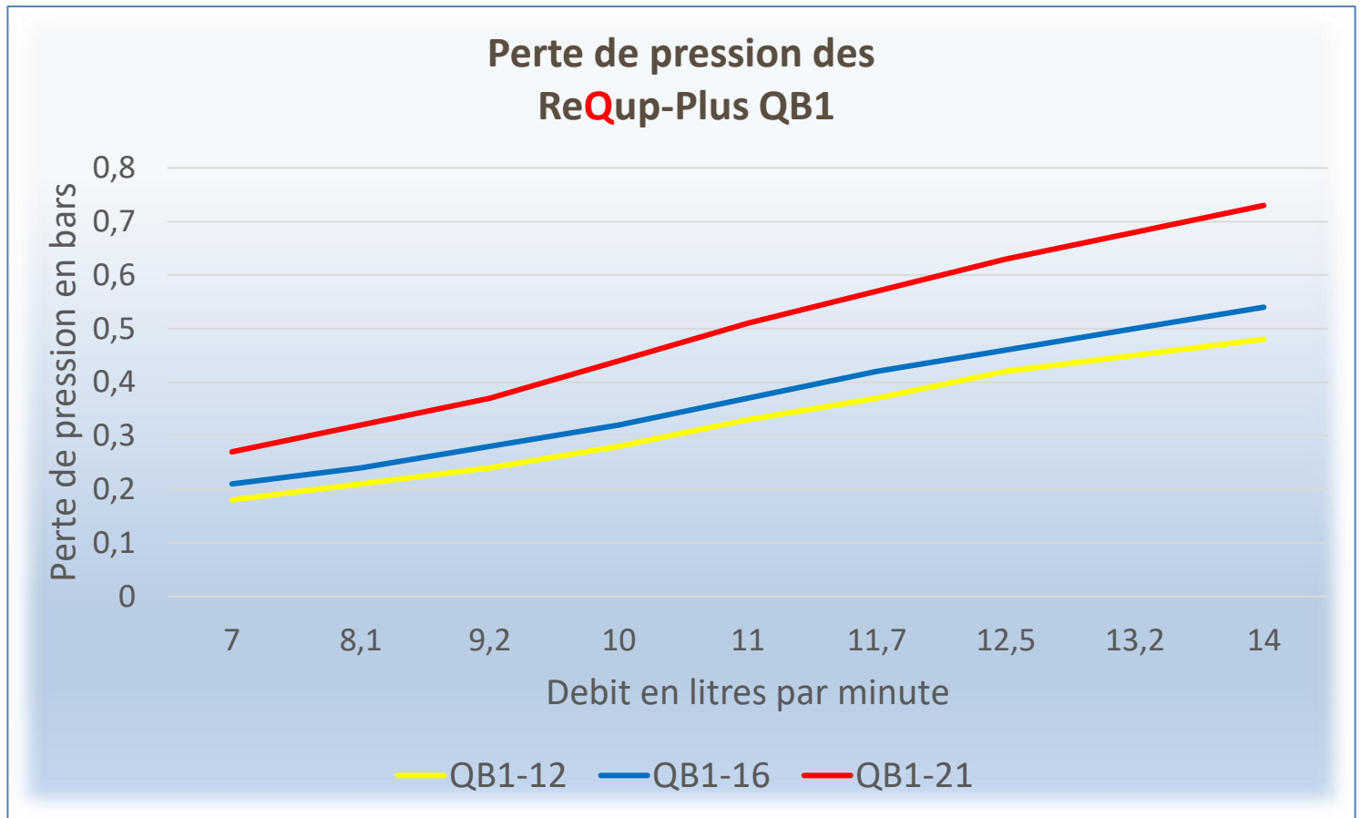
Fig. 7 Perte de pression QB1
