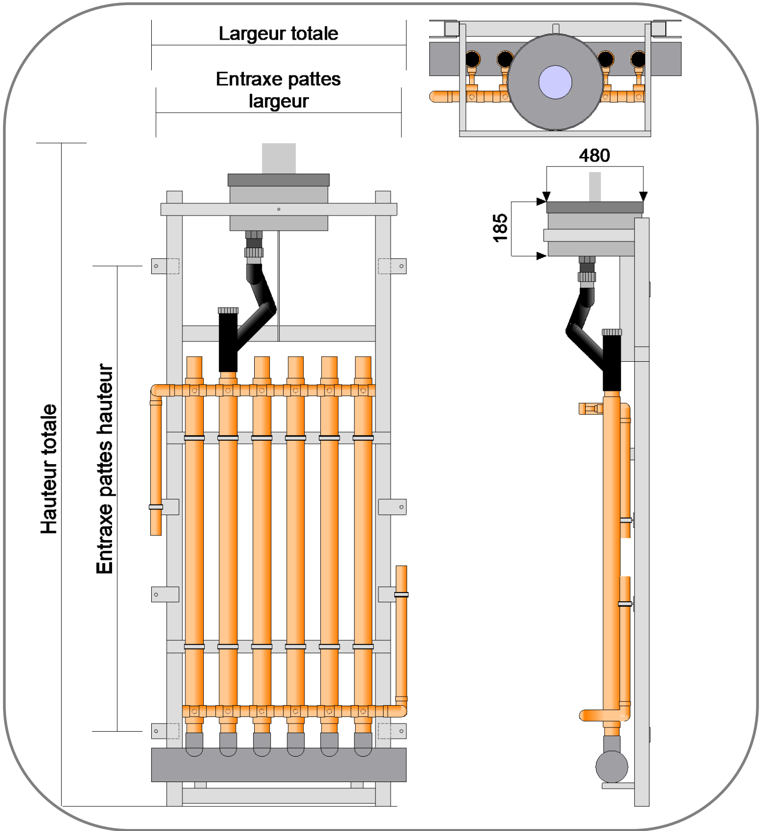
Fig. 6 Schéma de principe ReQup-Plus Multi
